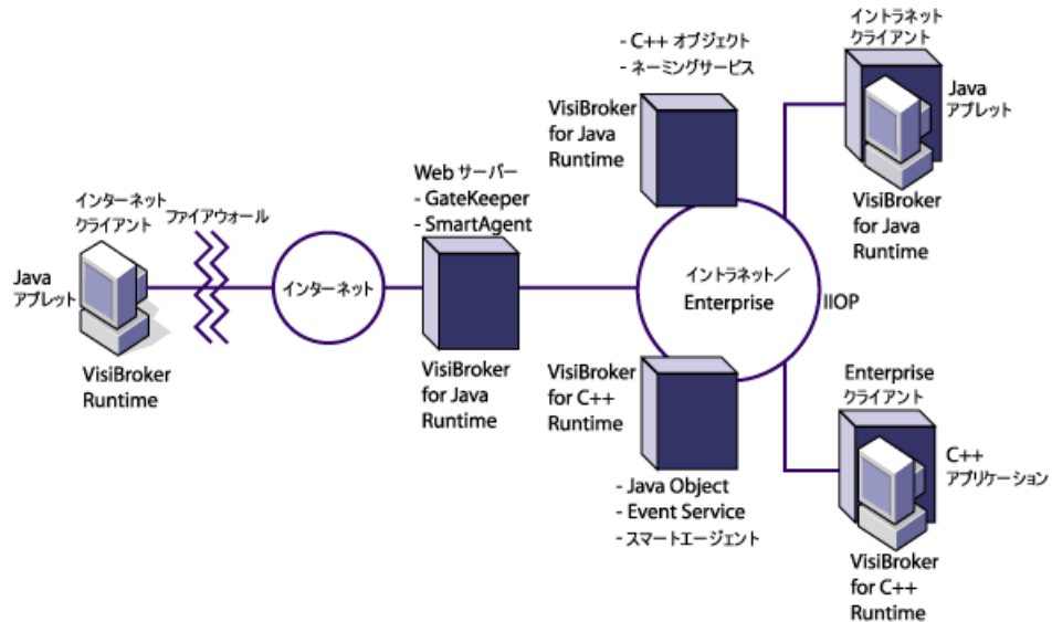
図 1.2 VisiBroker のアーキテクチャ
