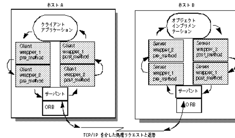
図 25.2 複数の型なしオブジェクトラッパー
