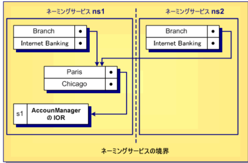
図 15.3 複数のアクセス階層を含むネーミングコンテキスト
