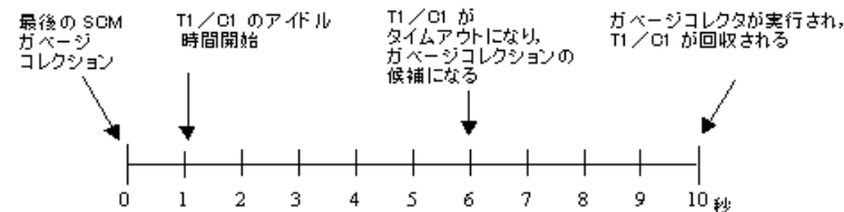
図 9.9 ORB GC によるリソースの回収
