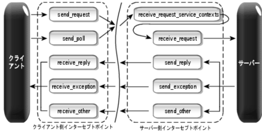
図 23.2 要求インターセプトポイント
