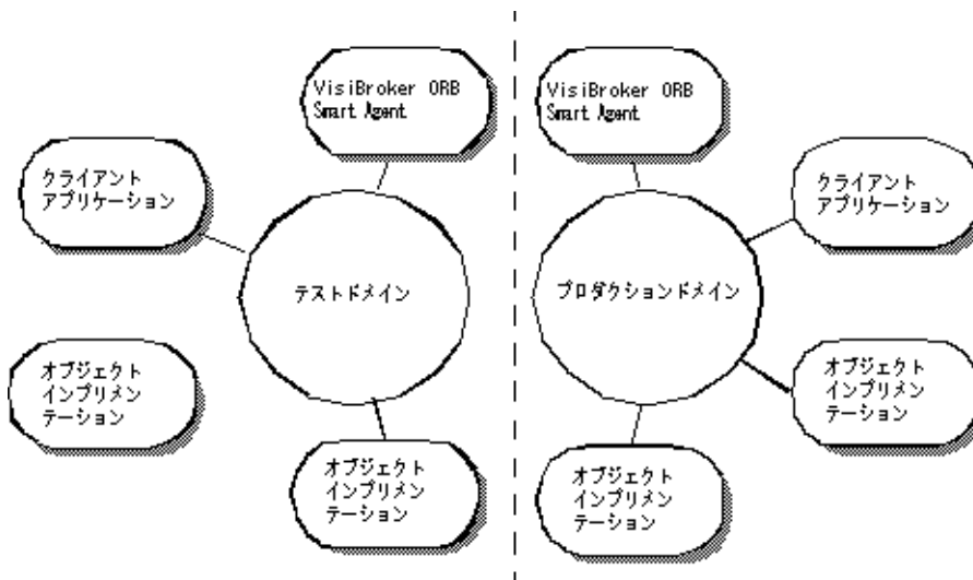
図 13.1 異なる VisiBroker ORB ドメインの同時実行
