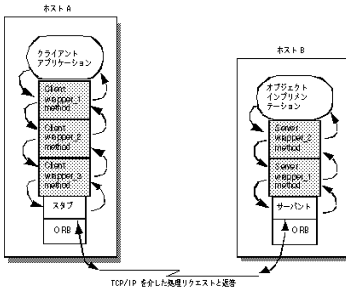
図 25.4 登録された複数の型付きオブジェクトラッパー
