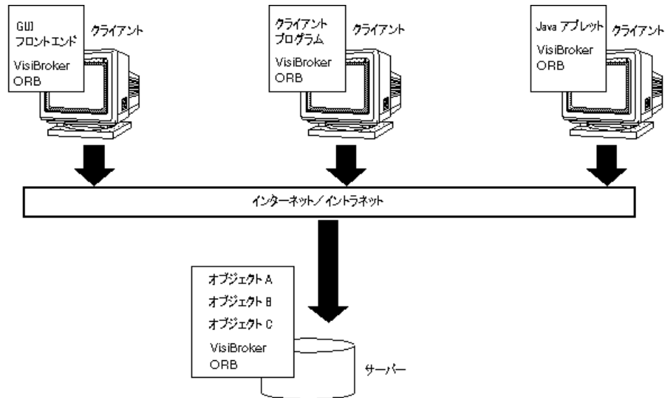
図 2.2 VisiBroker ORB を使ってデプロイメントされるクライアントプログラムとサーバープログラム
