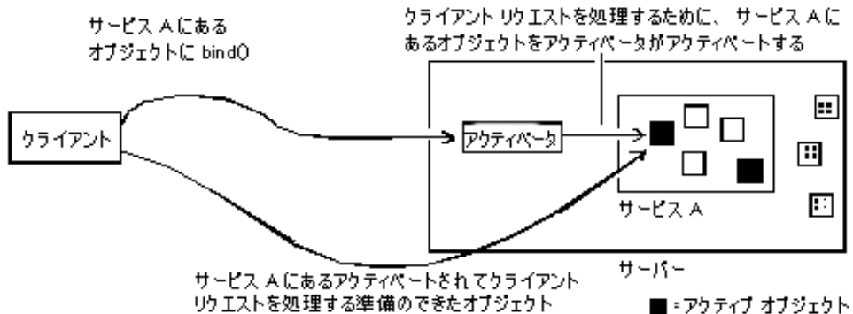
図 33.1 サービスのアクティブ化の遅延プロセス
