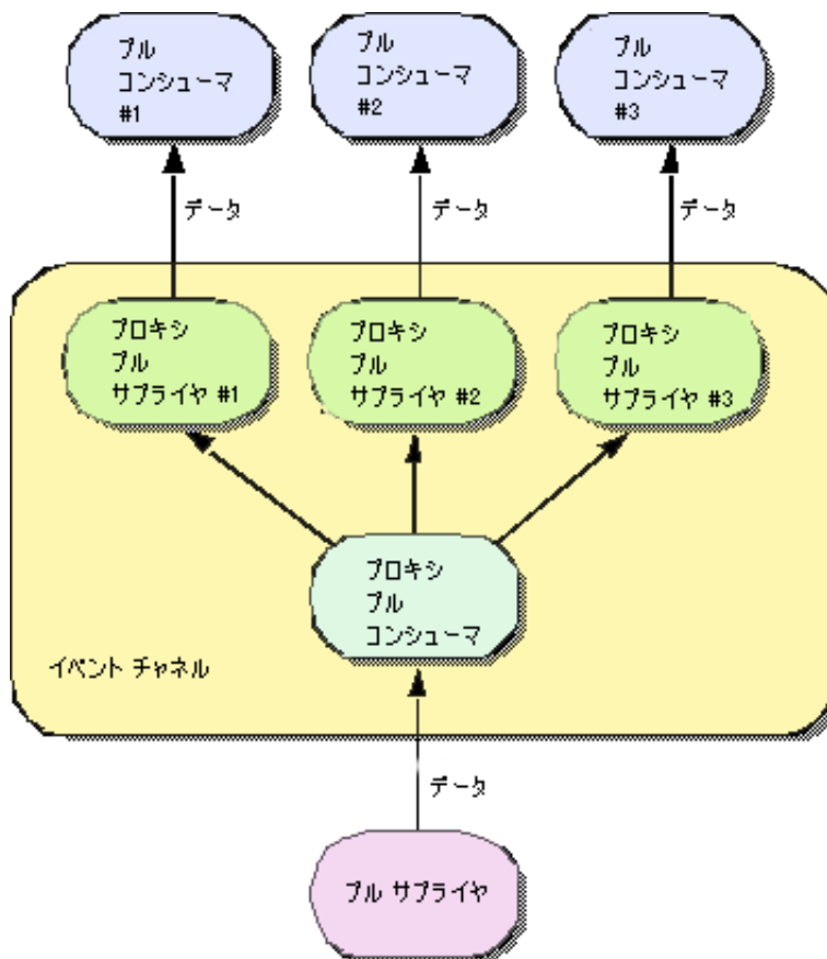
図 16.4 プルモデル
