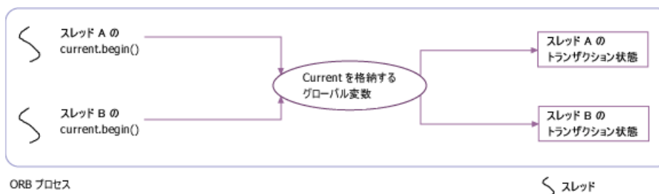
図 7.2 グローバルな Current オブジェクトを使ってプロセス内の複数のスレッドにまたがるトランザクションを開始する方法
