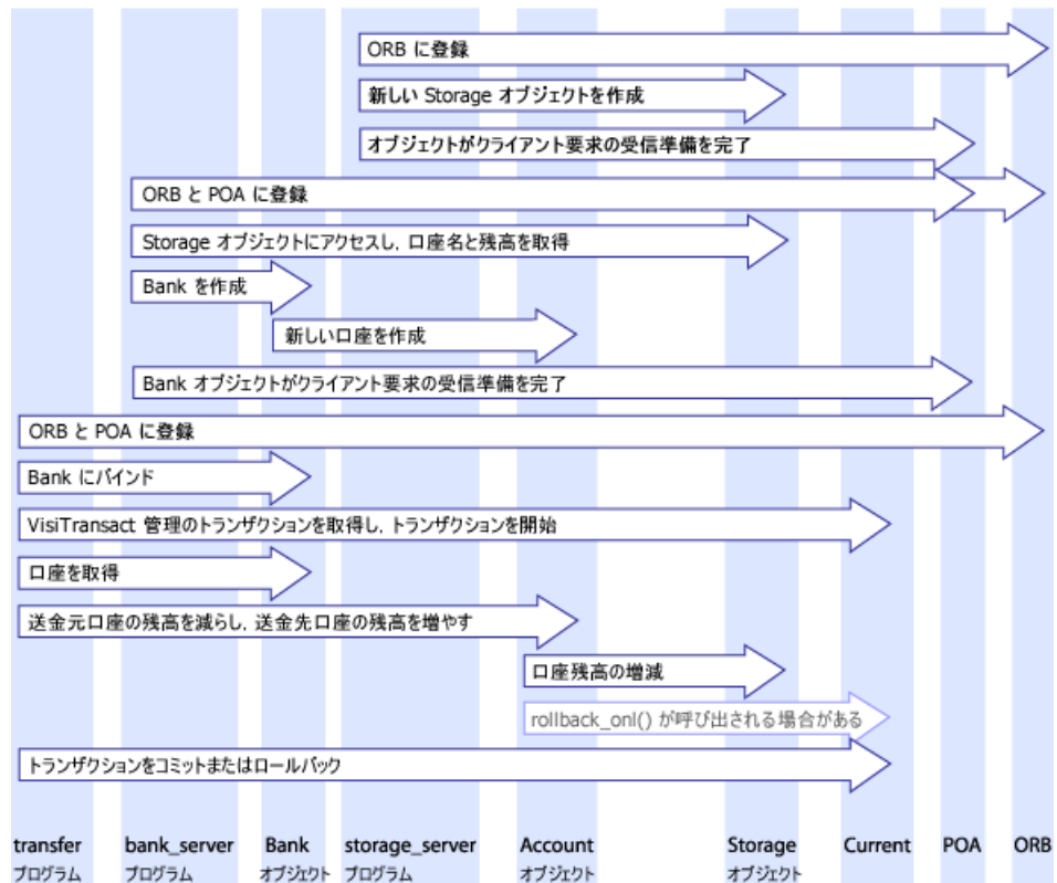
図 4.2 次は、クイックスタートサンプルでアプリケーションが行う呼び出しを図で表したものです。
