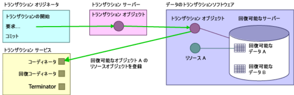
図 10.2 回復可能なデータのためのリソースオブジェクトを登録する
