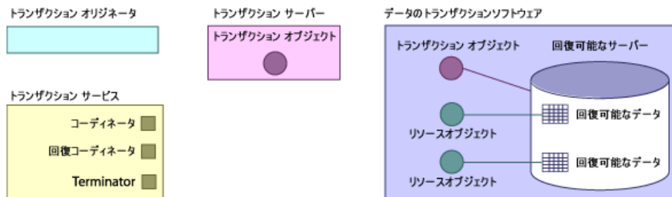
図 10.1 2 フェーズコミットに関するオブジェクト
