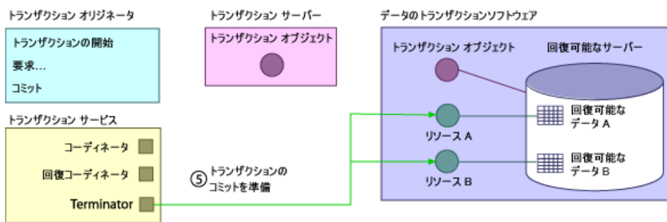
図 10.4 Terminator はリソースオブジェクトにトランザクションのコミットを準備するように要請する
