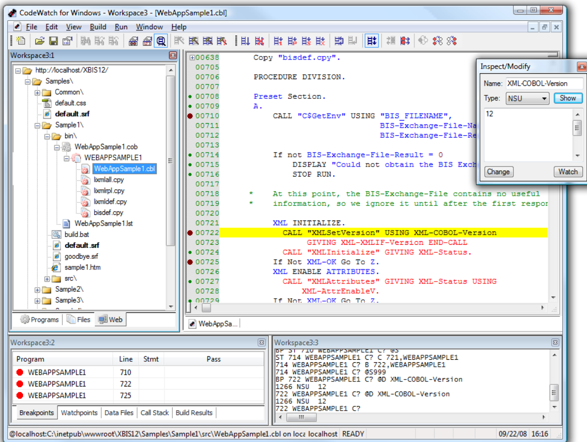
Figure 1. CodeWatch for BIS
