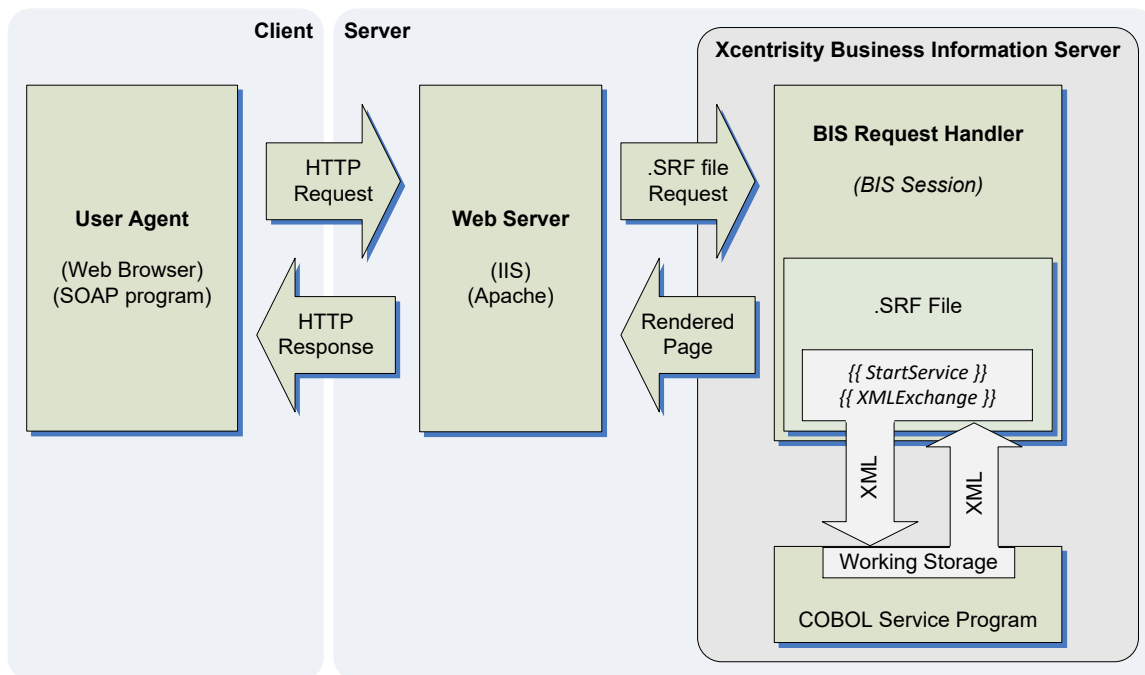
Figure 9. BIS Control Flow
